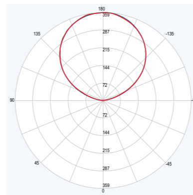
Standaard uitstraling pendelafstand 40-150cm.
