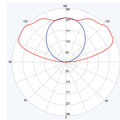
Extra wide beam voor lage plafonds. Pendelafstand 16-40cm
